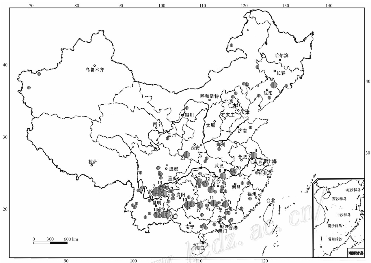
图2 中国MVT矿床分布示意图
