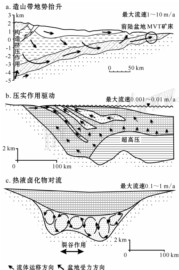
图 3 MVT 铅锌矿床流体运移模式
