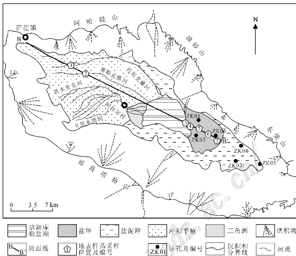
图 1 尕斯库勒盐湖钻孔和地表沉积物采样点分布图(底图改自刘成林等, 2013)
