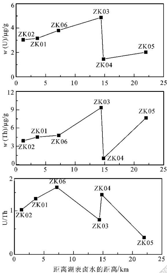
图3 奈斯库勒盐湖各钻孔 w(U) 、 w(\text{Th}) 、 U/\text{Th} 值随湖表卤水距离的变化
