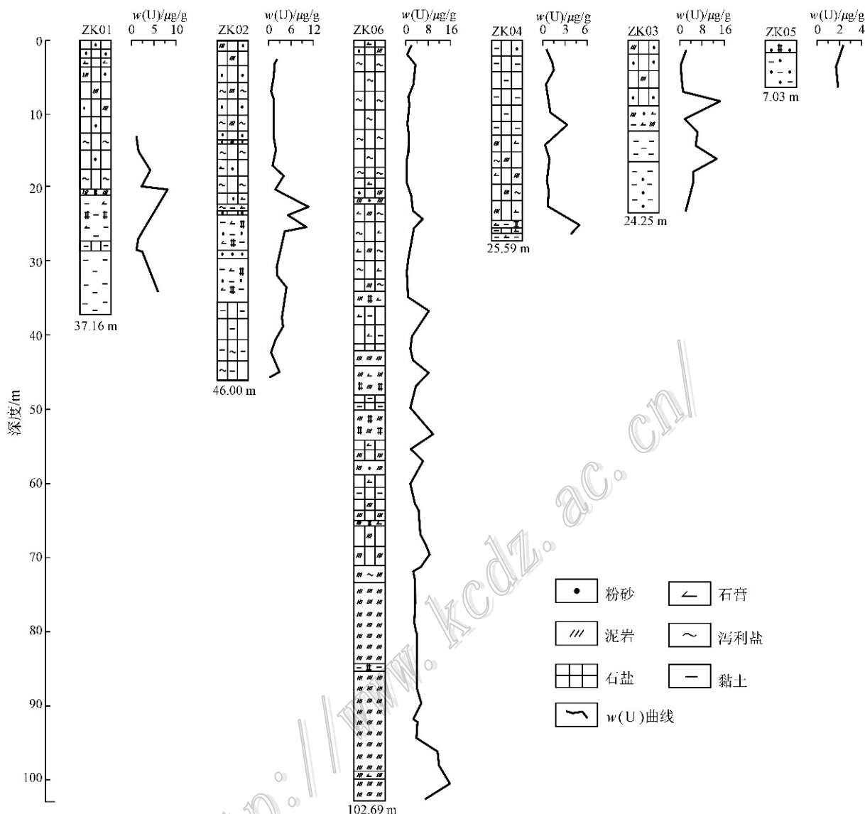
图 4 杂斯库勒盐湖钻孔沉积物中铀的分布特征
