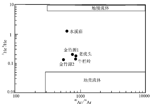
图3 成矿流体的 ^3\text{He}/^4\text{He} - ^{40}\text{Ar}/^{36}\text{Ar} 图解 (据丰成友等, 2006 修改)
