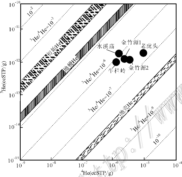
图 2 成矿流体的 ^3\text{He}-^4\text{He} 同位素演化图解 (据胡瑞忠等,1999 修改)
