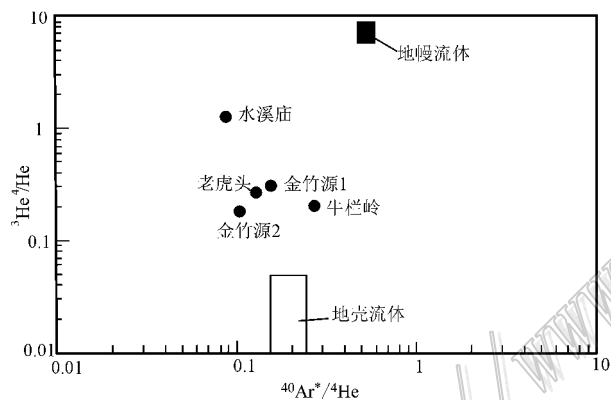
图4 成矿流体的 ^3\text{He}/^4\text{He} - ^{40}\text{Ar}^*/^4\text{He} 图解 (据胡瑞忠等, 1997 修改)
