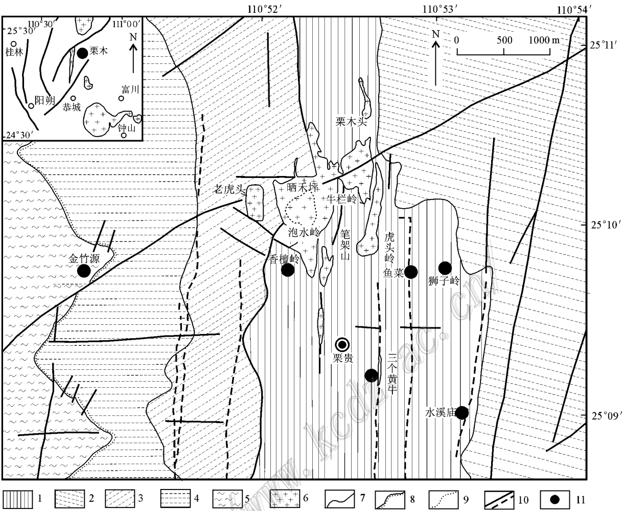
图 1 栗木矿田地质略图(据覃宗光等,2008 修改)
