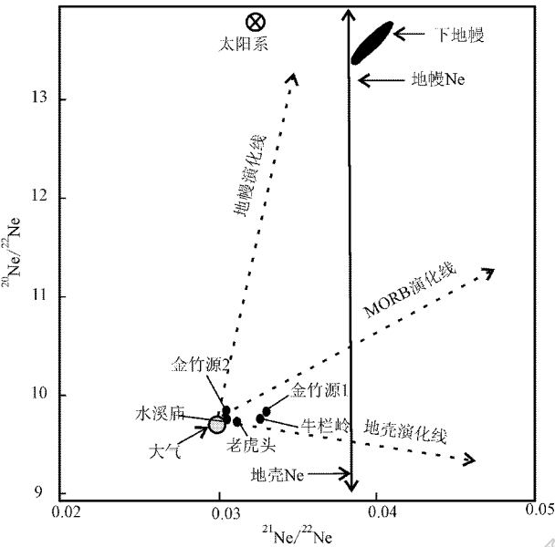
图 5 栗木矿田成矿流体 ^{20}\text{Ne}/^{22}\text{Ne} - ^{21}\text{Ne}/^{22}\text{Ne} 图解 (据 Hilton et al., 2002 修改)
