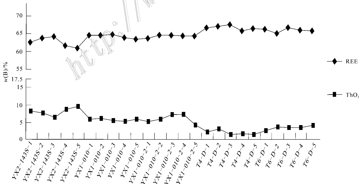
图 7 波孜果尔碱性岩中独居石中 ThO 2 和 REE 化学成分变化图解 Fig. 7 Diagrams of ThO 2 and REE of monazite from Boziguoer alkali rocks
