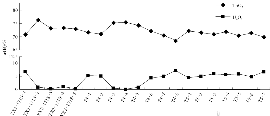
图 6 波孜果尔碱性岩中钍石中 ThO 2 和 U 2 O 5 化学成分变化图解 Fig. 6 Diagrams of ThO 2 and U 2 O 5 of thorite from Boziguoer alkali rocks
