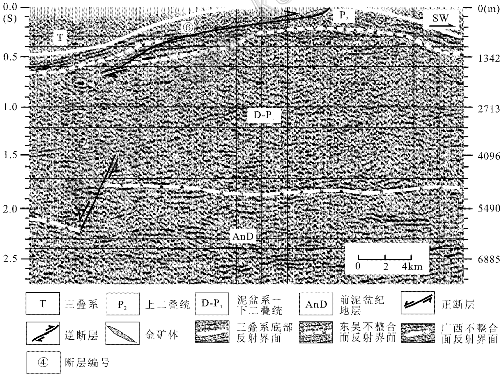
图 3 大丫口金矿地震偏移剖面解释图
