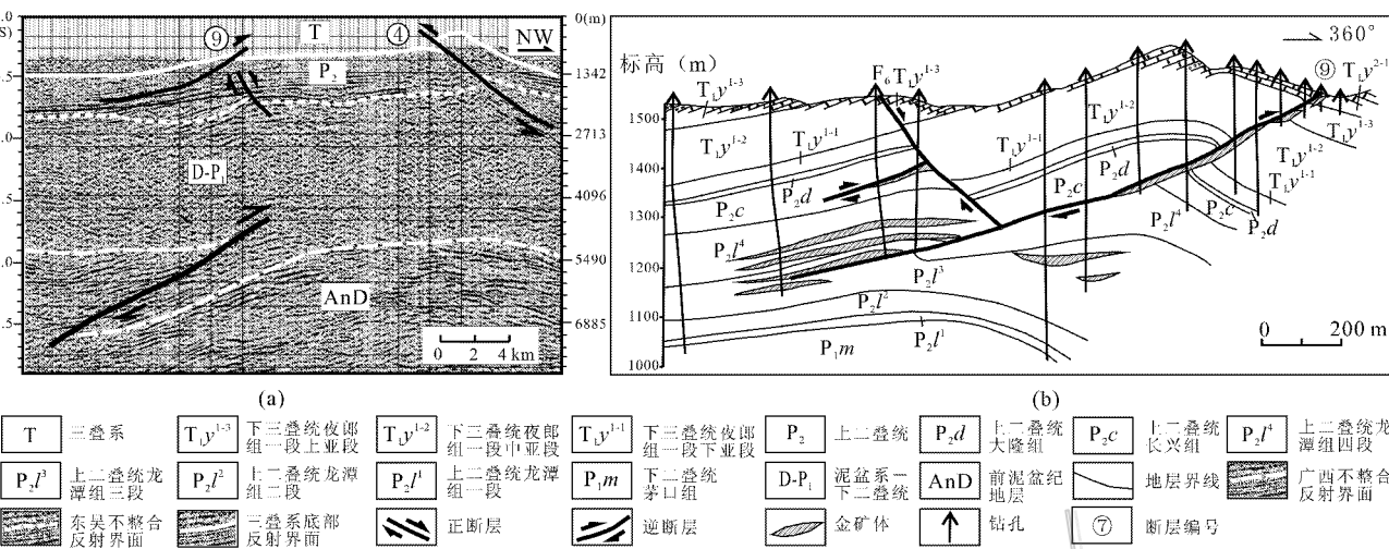
图 2 灰家堡矿田地质-地震对比图(右图据王砚耕,1994 资料修改)
