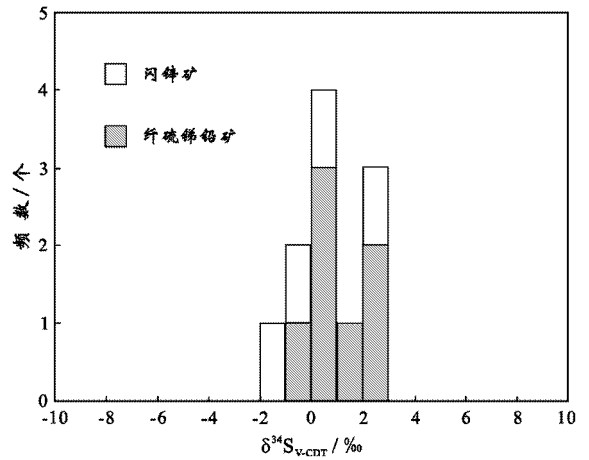
图 12 拉诺玛矿床内矿石硫化物的硫同位素组成
