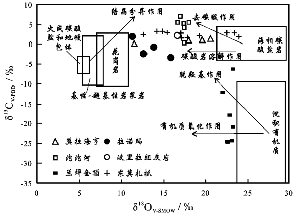
图 11 拉诺玛矿床内热液方解石的碳、氧同位素组成典型岩石类型的碳、氧同位素组成分布及三江铅锌矿带沱沱河盆地、囊谦盆地、东莫扎抓、莫拉海亨、铅锌矿床、兰坪金顶铅锌矿床的资料据刘家军等 2004 及 He et al. 2009
