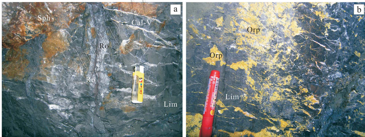
图4 拉诺玛矿床典型矿石矿物产出照片
