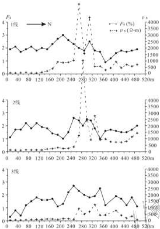
图 1 伊尔曼得金矿床激电剖面图
