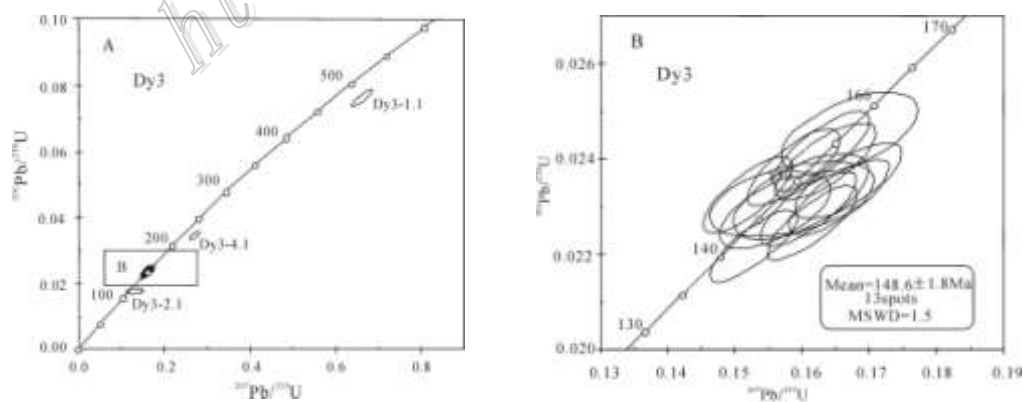
图 1 东源花岗斑岩体中锆石 SHRIMP U-Pb 年龄谱和图
