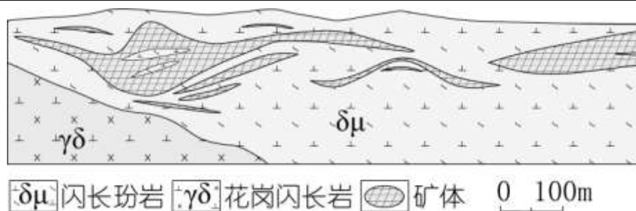
图1 宁芜盆地和尚桥铁矿床剖面 (据宁芜研究项目编写小组, 1977 修改)
