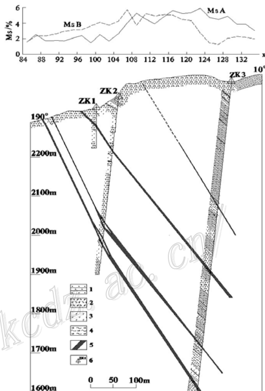
图 5 56 号勘探线综合剖面图
