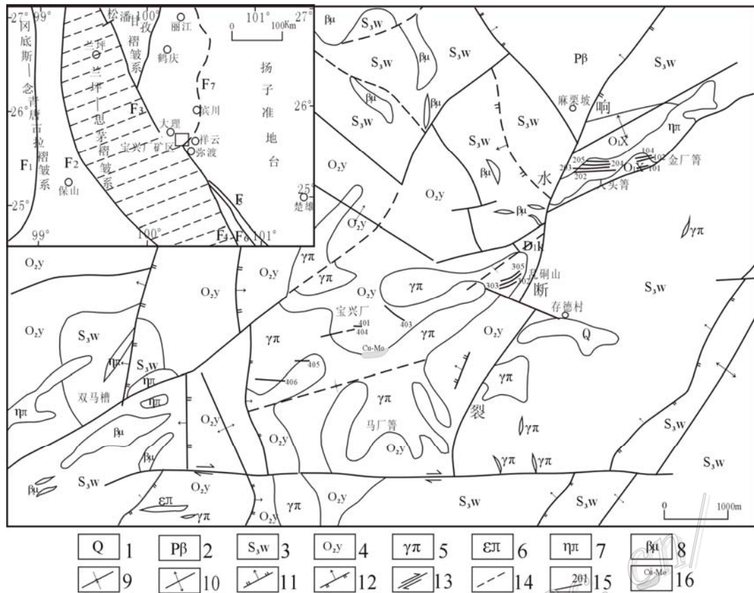
图 1 宝兴厂矿区地质图
