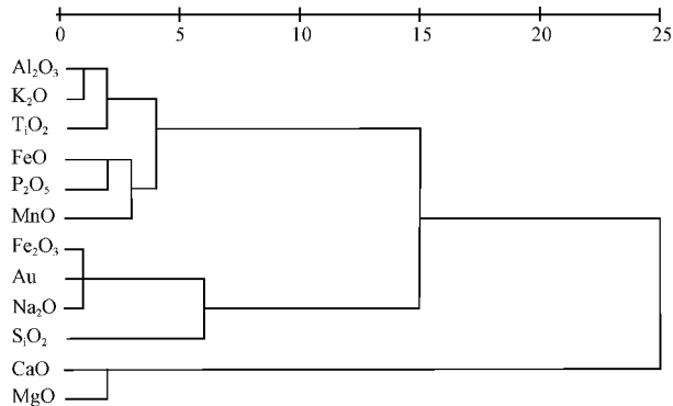
图 3 大庄子金矿床常量元素与金元素 R 型分层聚类图
