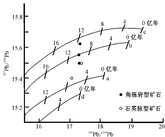
图6 大庄子金矿床铅同位素构造模式图
