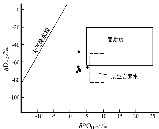
图8 大庄子金矿 \delta D_{H_2O} - \delta^{18}O_{H_2O} 关系图
