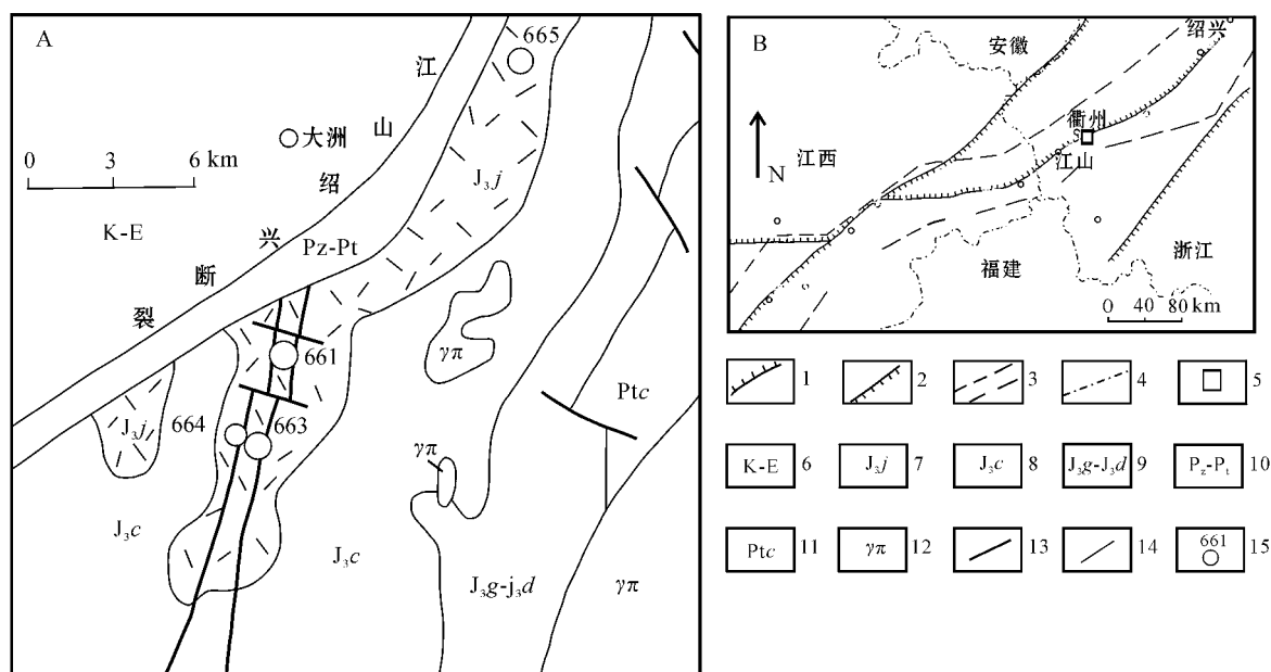
图 1 661 矿床区域地质略图(A)及研究区大地构造位置略图(B)(据张星蒲,1999 和毛孟才,2004 修改)
