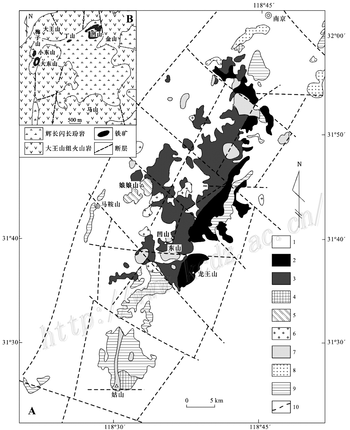
图 1 A. 宁芜盆地地质简图; B. 凹山和东山铁矿地质简图( 据宁芜研究项目编写小组, 1978 )
