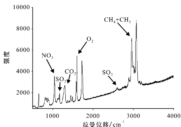
图 4 石英中流体包裹体气液相成分的激光拉曼谱图
