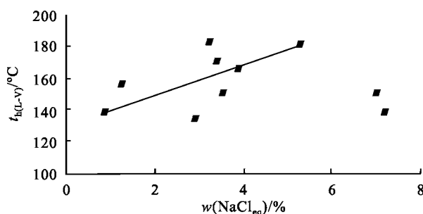
图 7 世代Ⅲ包裹体盐度-均一温度图
