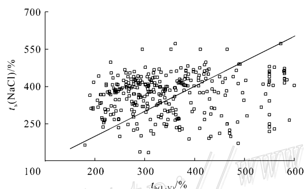
图 5 包裹体子矿物熔化温度-气泡消失温度图
