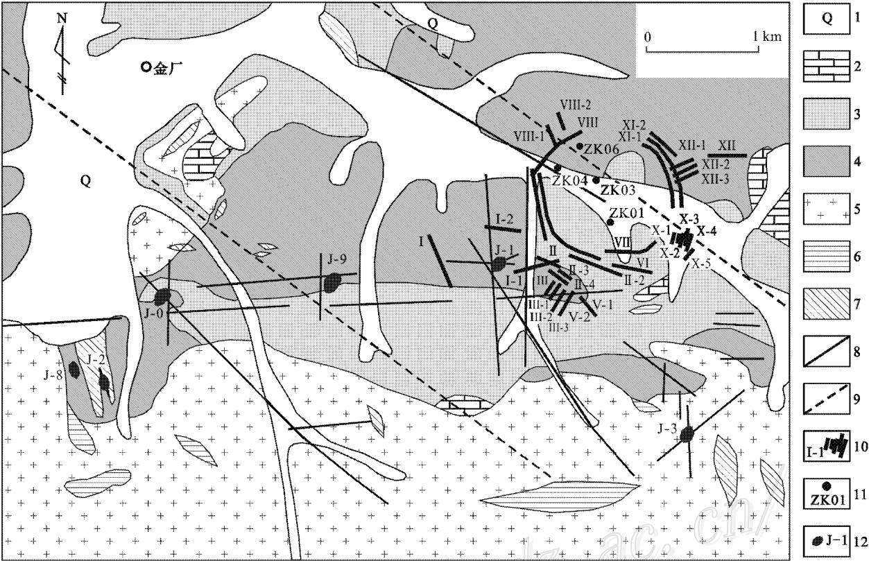
图 1 金厂矿区地质简图(底图据陈锦荣等 ① 2002 修改)
