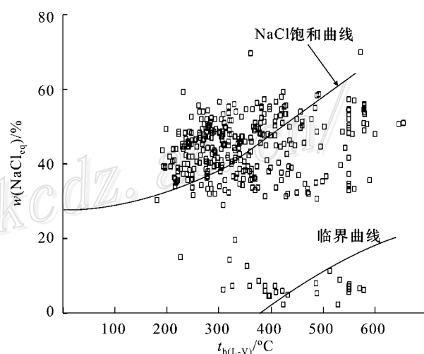
图 6 包裹体盐度-均一温度图(底图据 Calagari 2004)
