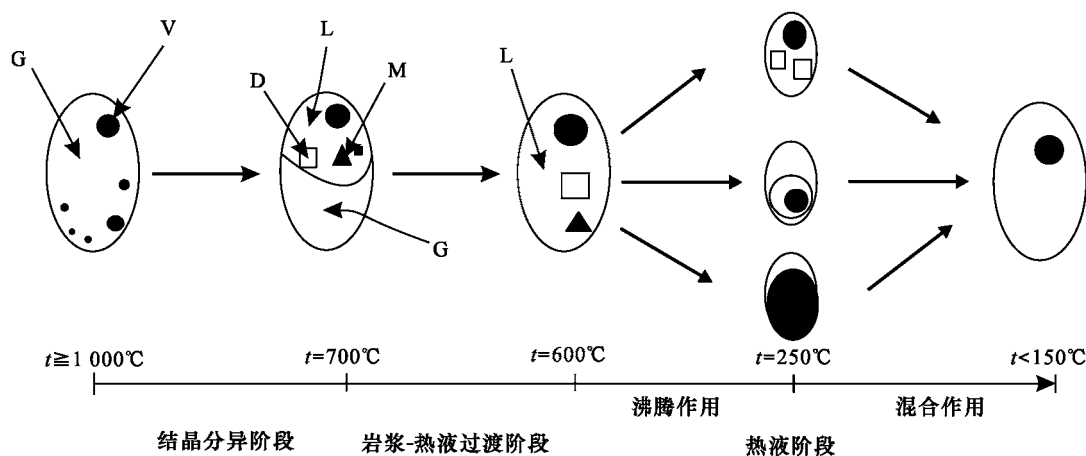
图 8 岩浆结晶分异示意图
