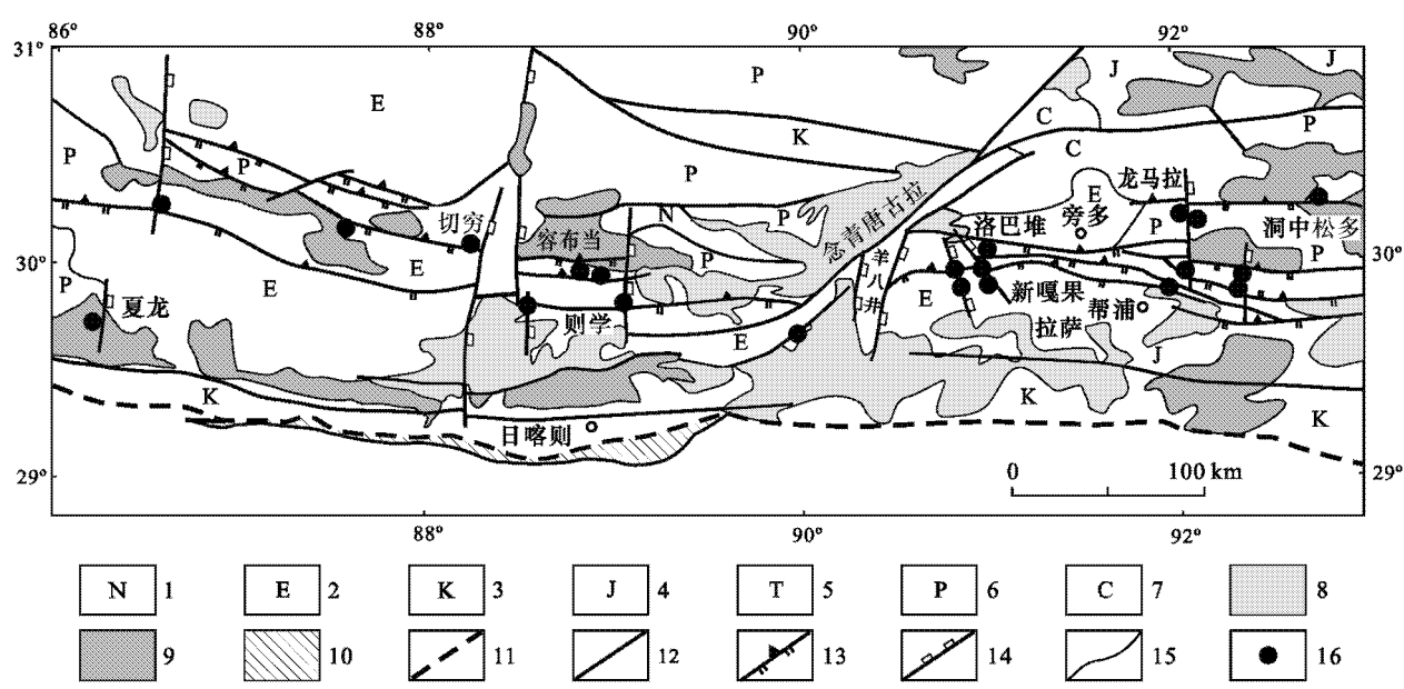
图 1 冈底斯构造-岩浆带的构造格架及银多金属矿床的分布 1—新近系 2—古近系 3—白垩系 4—侏罗系 5—三叠系 6—二叠系 7—石炭系 8—喜马拉雅期花岗岩 9—燕山期花岗岩 10—蛇绿岩 11—缝合带 12—断层 13—逆冲断裂 14—张性构造 15—地质界线 16—银多金属矿 Fig. 1 Tectonic framework of the Gangdese tectonic belt , showing distribution of silver-polymetallic deposits 1—Neogene 2—Paleogene 3—Cretaceous 4—Jurassic 5—Triassic 6—Permian 7—Carboniferous 8—Himalayan granite 9—Yanshanian granite 10—Ophiolite 11—Suture zone 12—Fault 13—Thrust fault 14—Tension fault 15—Geological boundary 16—Silver-polymetallic deposit
