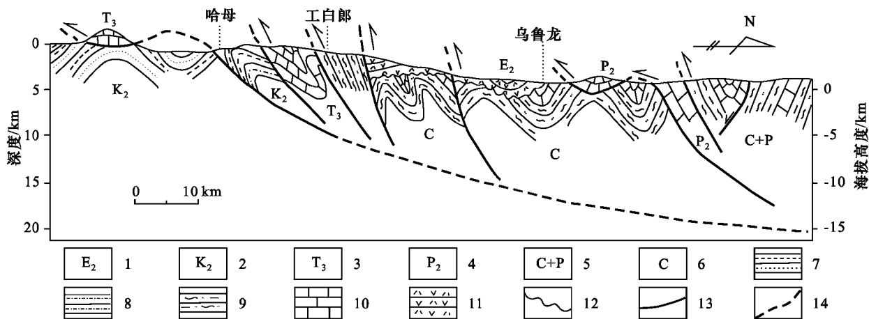
图 2 冈底斯带旁多逆冲系构造式样(据叶培盛, 2004)
