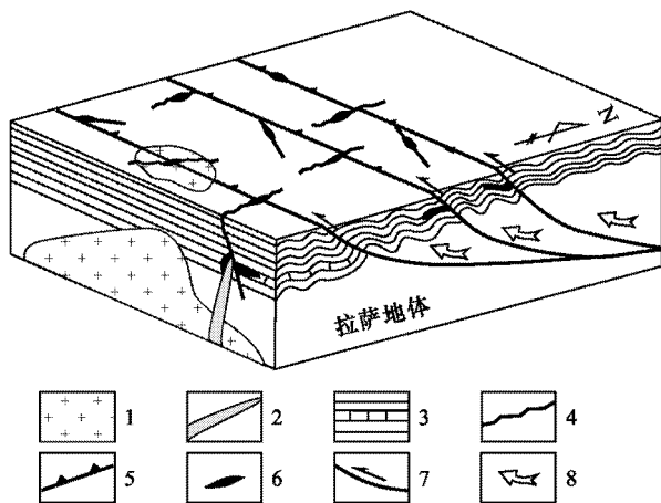
图 4 冈底斯银多金属矿化带成矿作用示意图
