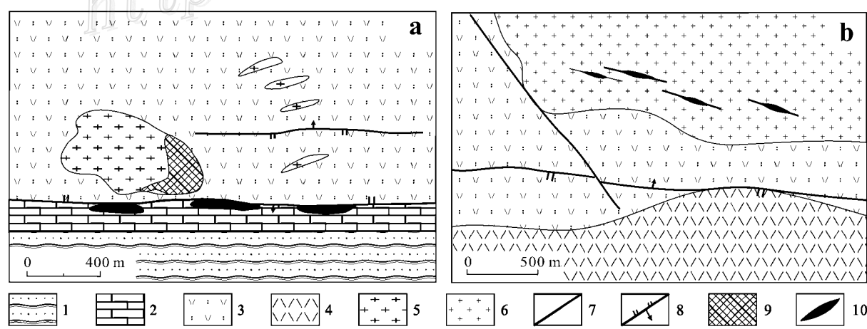
图 3 冈底斯银多金属矿化带帮浦矿床(a)和切穷矿床(b)地质略图
