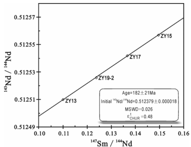
图 1 紫云石头寨二叠系古油藏裂缝充填方解石 Sm-Nd 等时线图
