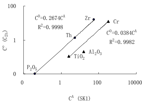
图 1 等浓度图解
