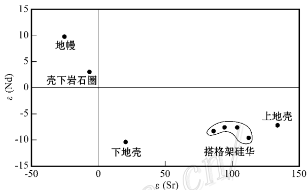
图 1 搭格架硅华 Sr 与 Nd 同位素图解
