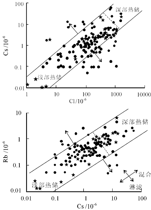
图 2 西藏热水中 Cs-Cl 及 Cs-Rb 相关图(侯增谦, 未刊资料)
