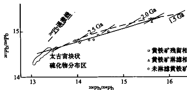
图 3 Temagami 矿山公路黄铁矿的淋滤相、残留相和未淋滤样品的铅同位素组成(据 Franklin et al., 1983)
