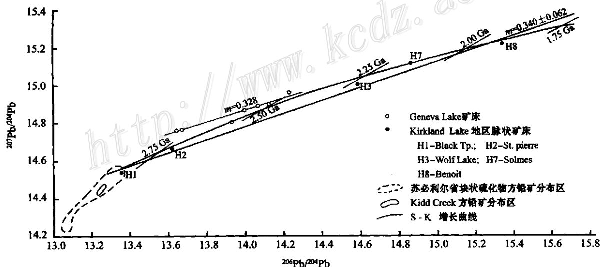
图 2 加拿大 Geneva Lake 火山岩型块状硫化物矿床和 Kirkland Lake 地区脉状硫化物矿床方铅矿的铅同位素组成 (据 Franklin et al., 1983)
