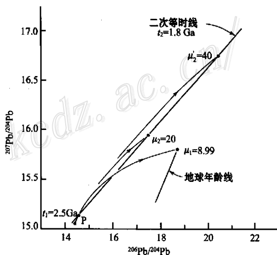
图 1 异常铅同位素演化图(据 Faure, 1977 修改)
