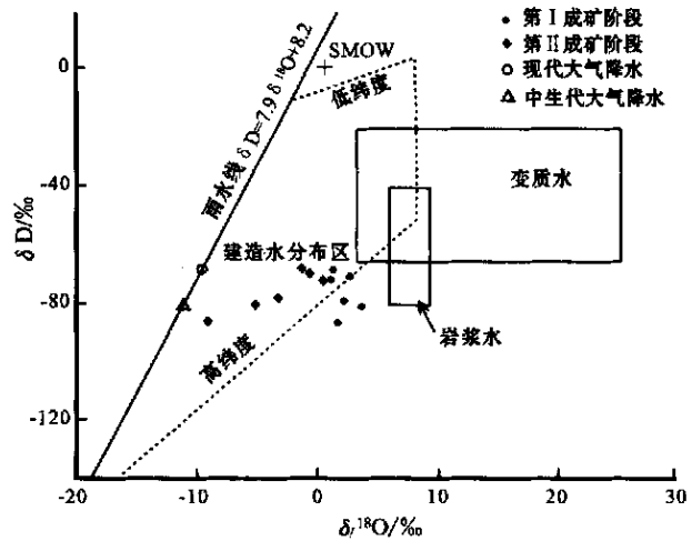
图 3 公峪金矿床成矿流体 \delta\text{D}-\delta^{18}\text{O}_{\text{H}_2\text{O}} 图解
