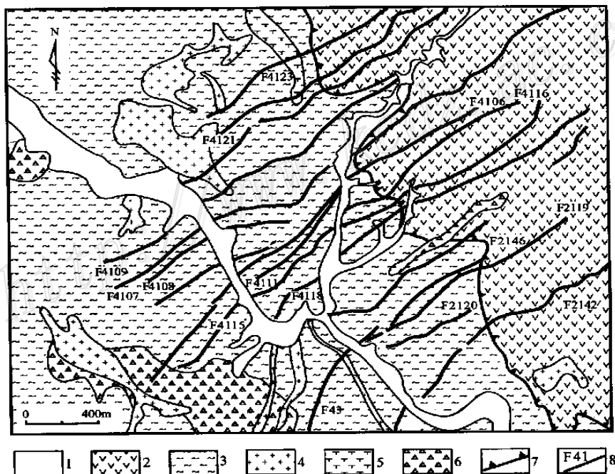
图 2 公峪矿区地质简图
