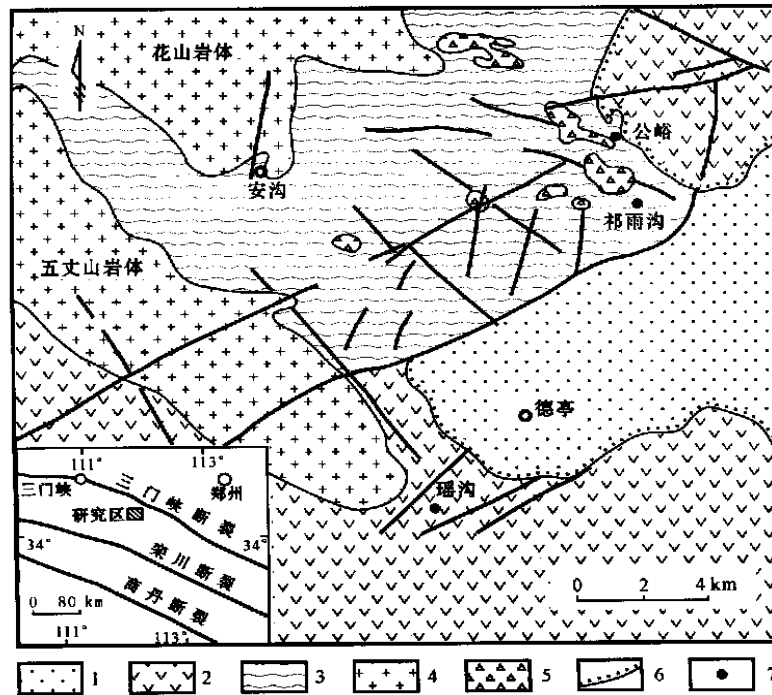
图 1 熊耳山东南部地质略图
