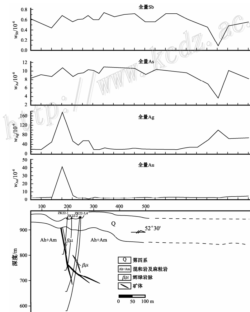
图 1 张全庄金矿土壤全量 Au, Ag, As, Sb 异常剖面图
