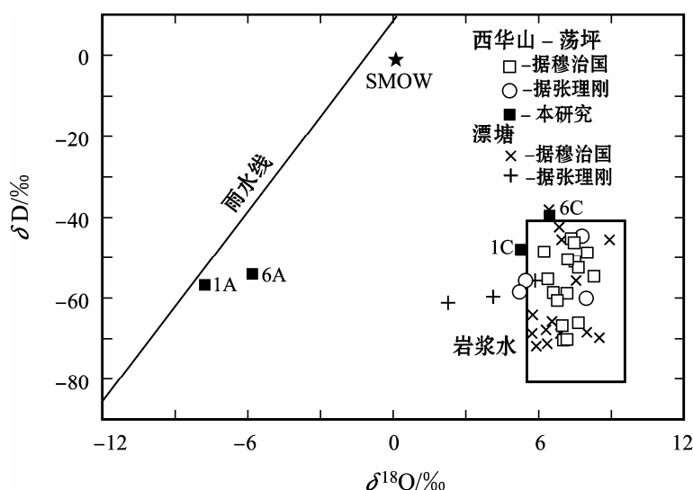
图2 西华山、荡坪和漂塘矿床成矿流体的 \delta^{18}\text{O} - \delta\text{D} 值图
