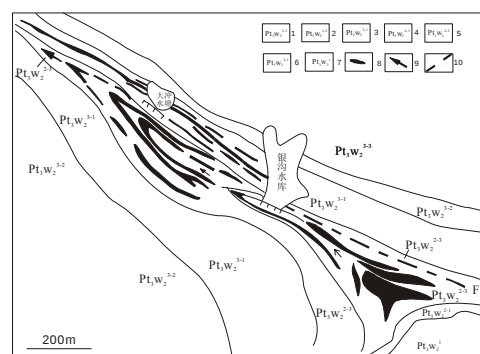
图 1 银洞坡金矿矿体分布示意图
