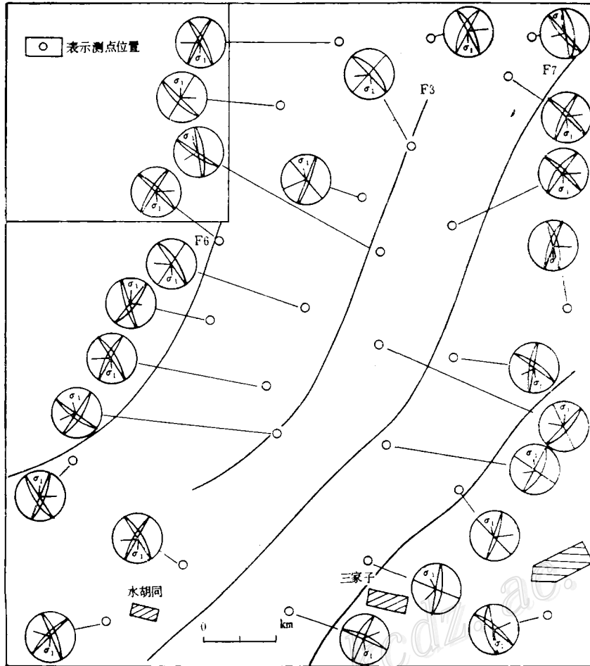
图 3 三家金矿区近SN向构造应力场主应力方向图 (小圆圈为测点位置线比例尺同图1)
