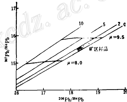
图 5 铅同位素组成坐标图
