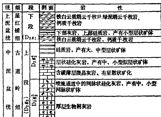
图1 凤太矿田铅锌矿床氧化硅产出层位综合示意图
