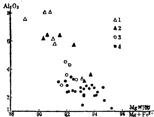
图 6 原生单斜辉石和新生单斜辉石的 \text{Al}_2\text{O}_3 和 \text{Mg} \times 100 / (\text{Mg} + \text{Fe}^{2+}) 相关图
