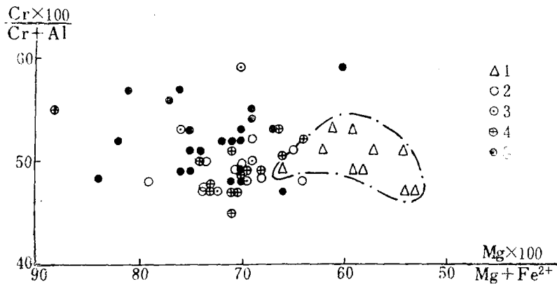
图 7 矿石及近矿纯橄岩中铬尖晶石的 \text{Cr} \times 100 / (\text{Cr} + \text{Al}) 和 \text{Mg} \times 100 / (\text{Mg} + \text{Fe}^{2+}) 相关图
