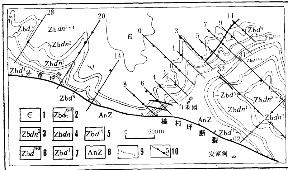
图 1 白果园矿区地质略图
