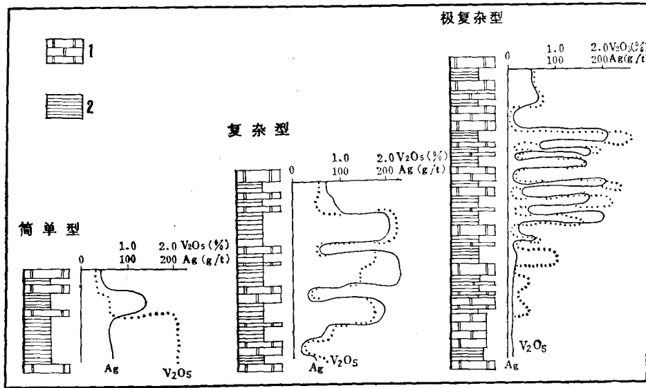
图 3 银钒矿层结构图
