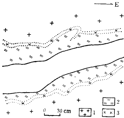
图5 形态受云英岩控制的红长石化岩 (594中段514石门957脉顶板) 1—斑状中粗粒黑云母花岗岩; 2—云母石英岩; 3—红长石化岩
