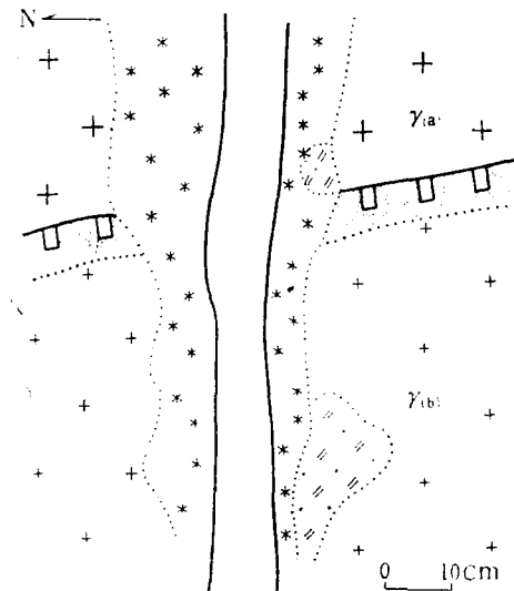
图 11 \gamma_{(a)} 和 \gamma_{(b)} 接触带上宽脉蚀变形态 (632中段503石门61脉北) (图例同图6、7、8)
