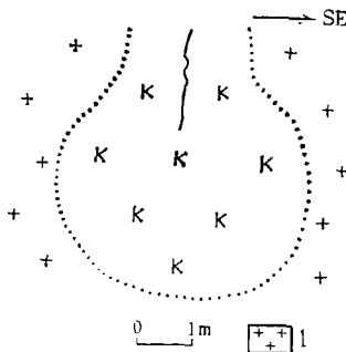
图7 矿脉根部红长石化岩 (431中段正巷北) 1—中粒花岗岩; 其它同图5
