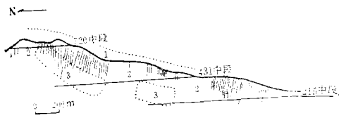
图1 红长石化分布综合剖面图
