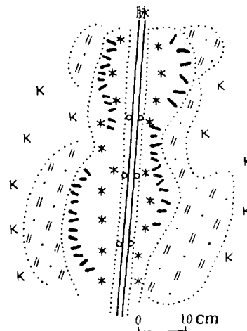
图6 内红长石化岩 (594中段91脉天井)
