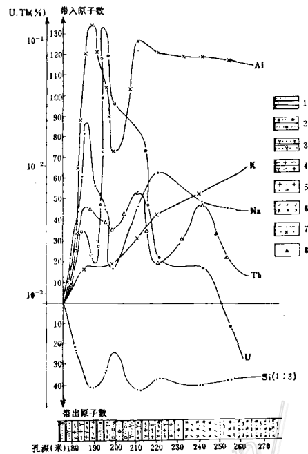
图3 钻孔柱状剖面中元素带入带出曲线 Fig. 3. Drill column indicating inward or outward migration of elements 1—石英岩；2—石英砾岩；3—混合质变质岩；4—斑杂状混合岩；5—均质混合岩和白色混合花岗岩；6—浅红色混合花岗岩；7—红色混合花岗岩；8—取样位置
