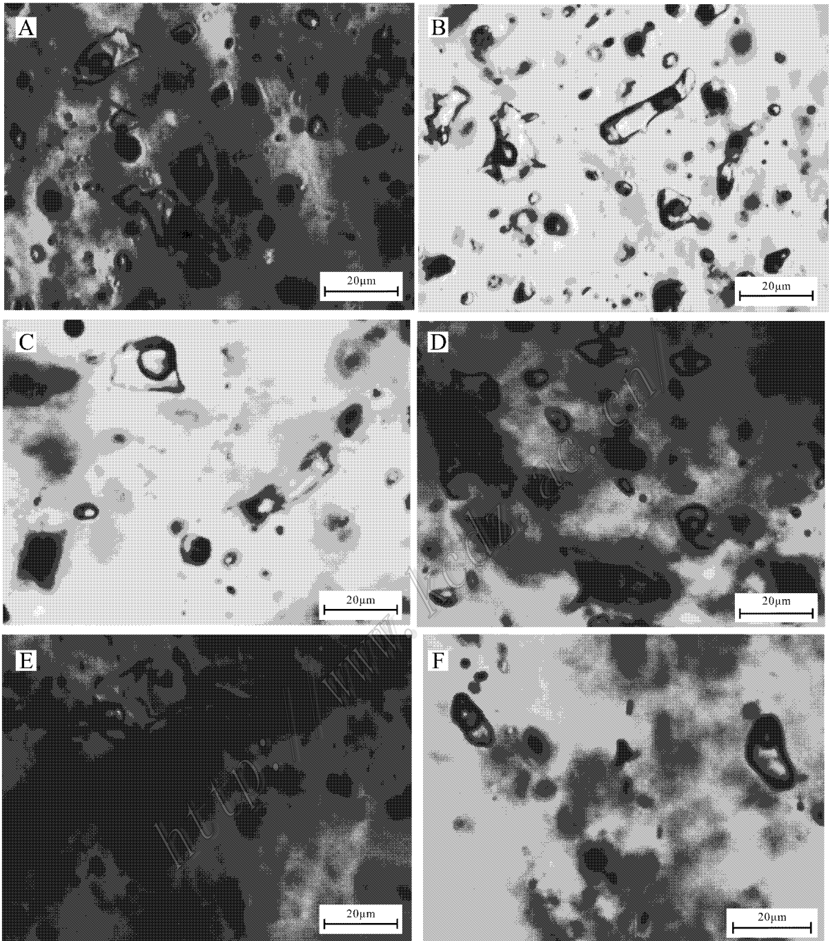
图4 老君山地区钼矿床流体包裹体显微照片
