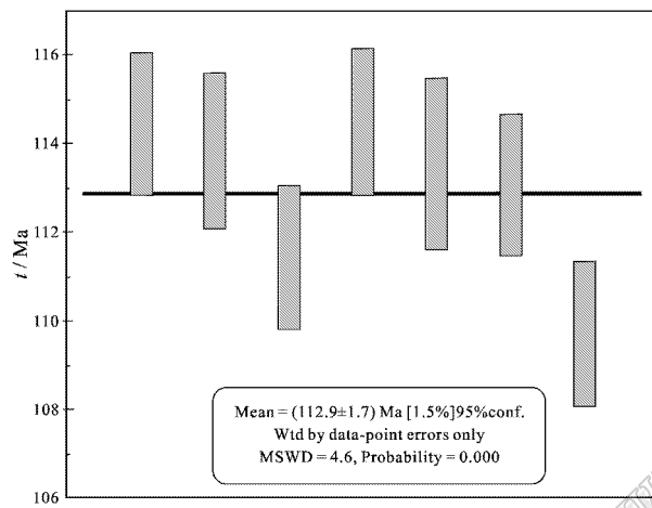
图 5 老君山地区钼矿中辉钼矿 Re-Os 模式年龄加权平均值
