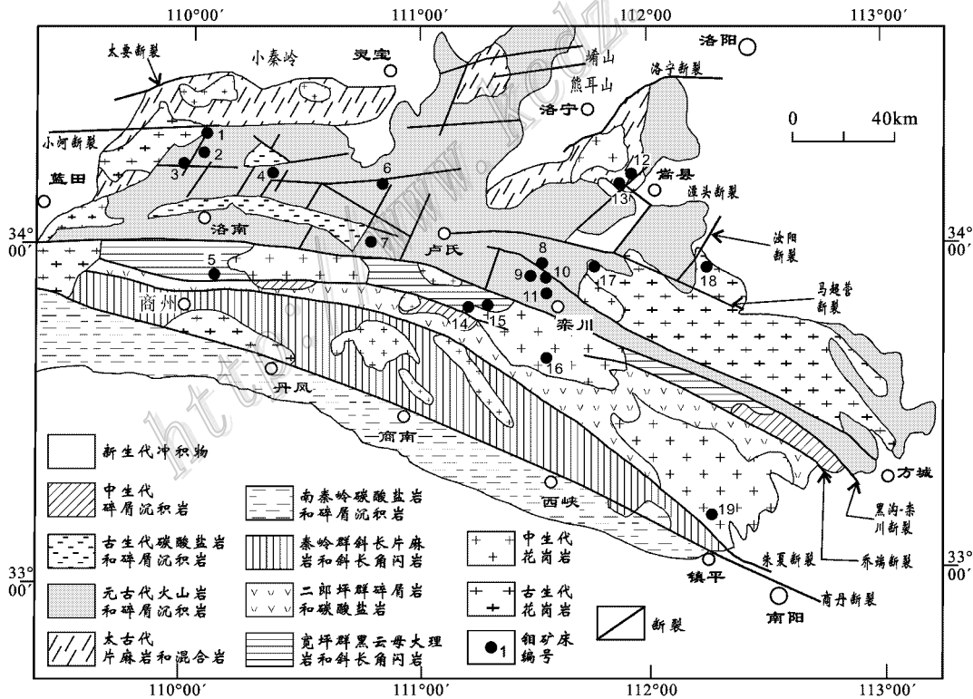
图 1 东秦岭钼矿带地质略图(据张正伟等,2007略改)
