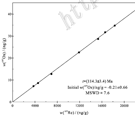
图 6 老君山地区钼矿中辉钼矿 Re-Os 同位素等时线
