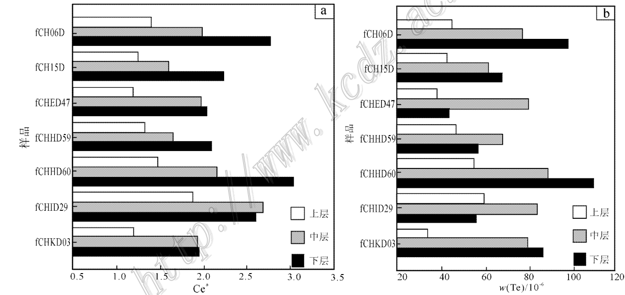
图 4 调查区结壳不同分层 Ce^* (a)和 \varpi(Te) (b)的变化及对比
